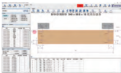
Modular UI
